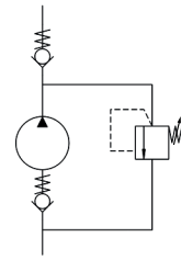
Schéma hydraulique
